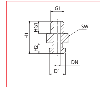
ANC-1,2-M5 ... ANC-8-1/4
