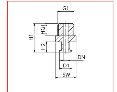
ANA-9-1/8 ... ANA41-1/4
