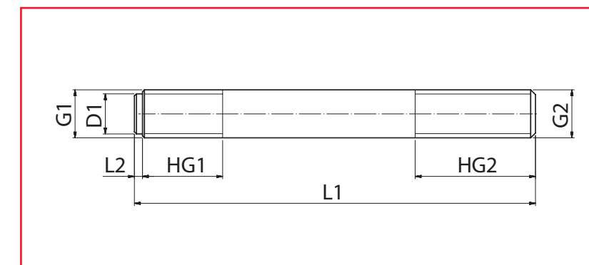
STG-M12x1 ... STG-M30x1,5
