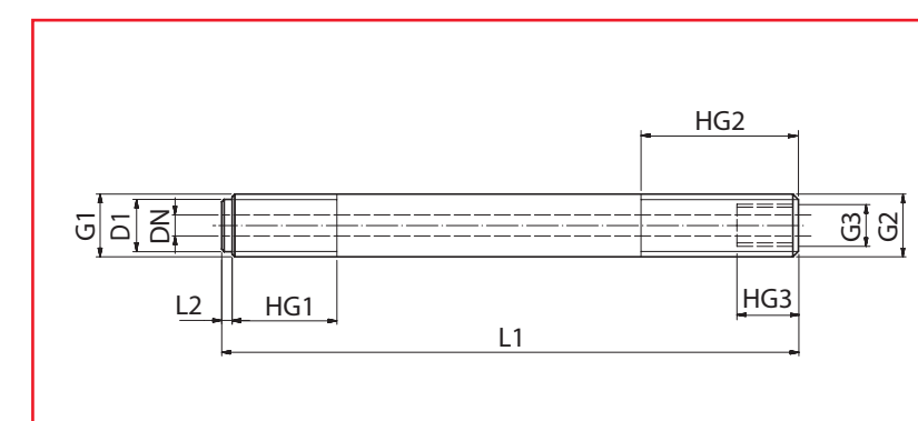
STI-M8x1 ... STI-M20x1,5
